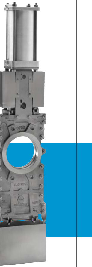
SER.30(TL) Through conduit K.G.V.
